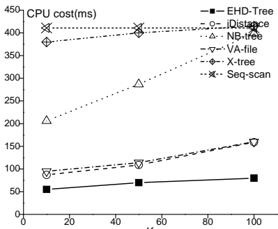
(a). real dataset
