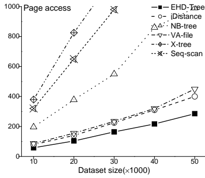
(a). real dataset
